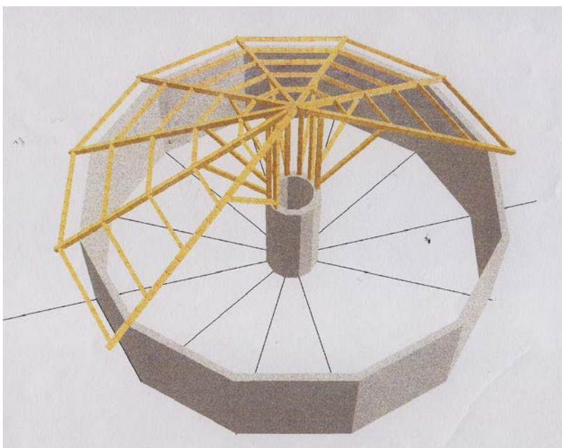
Dachstuhl des Bouldertempels
